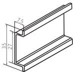
TH35-7.5 DIN Rail
